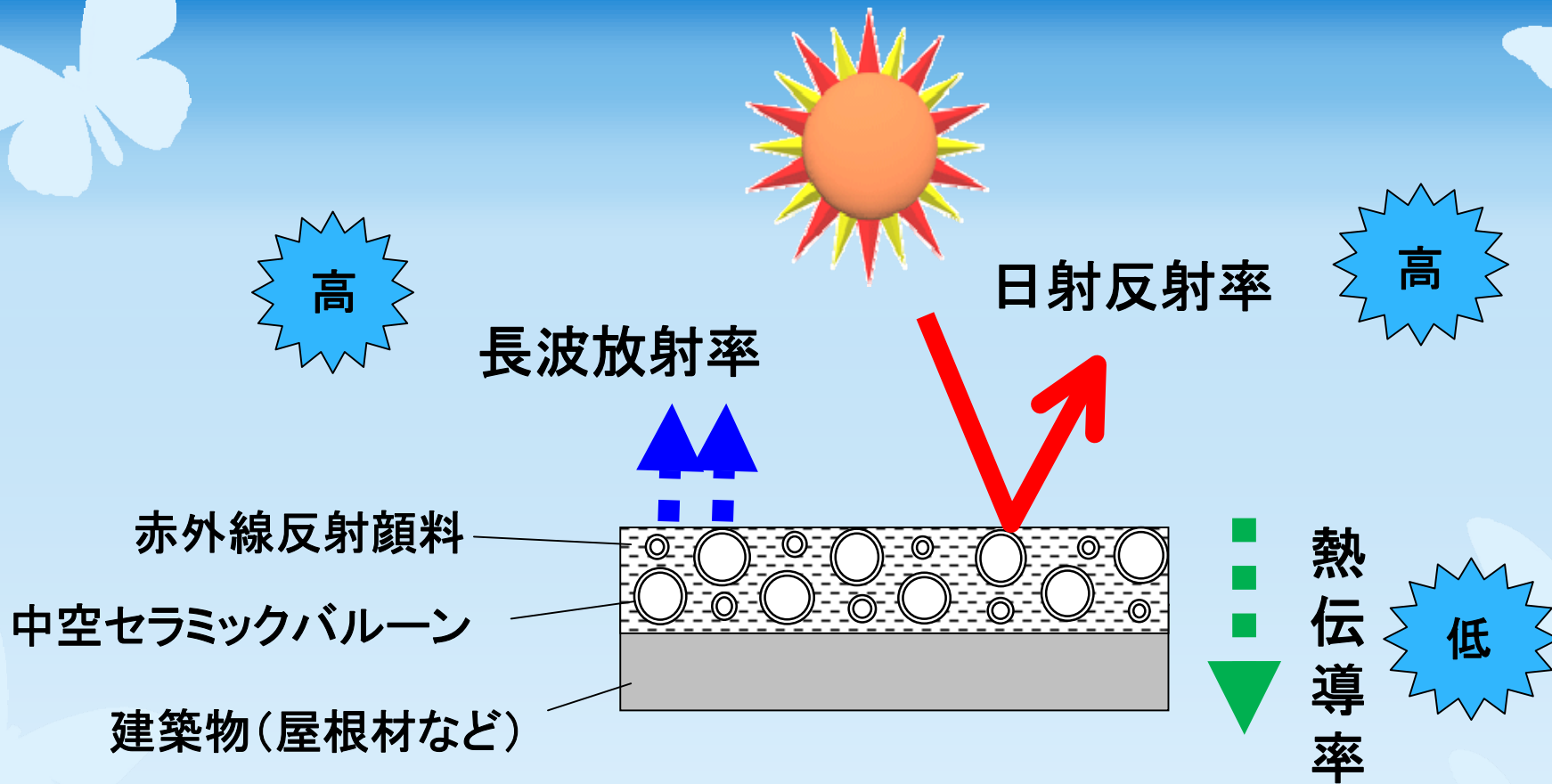
ミラクール塗膜の断面図
